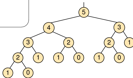
Diagram wywołań dla n=5:
