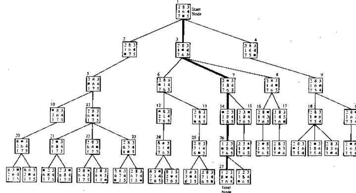
Diagram przedstawia fragment grafu przeszukiwania wszerz. Numery nad planszami (1–26) pokazują tu kolejność wyboru węzłów do ekspansji grafu.
