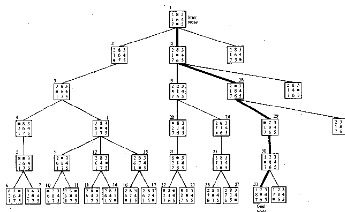
Fragment „przeciętnego” grafu przeszukiwania włąb z ograniczeniem głębokości do 5. Numery węzłów pokazują kolejność wyboru węzłów do ekspansji grafu.
